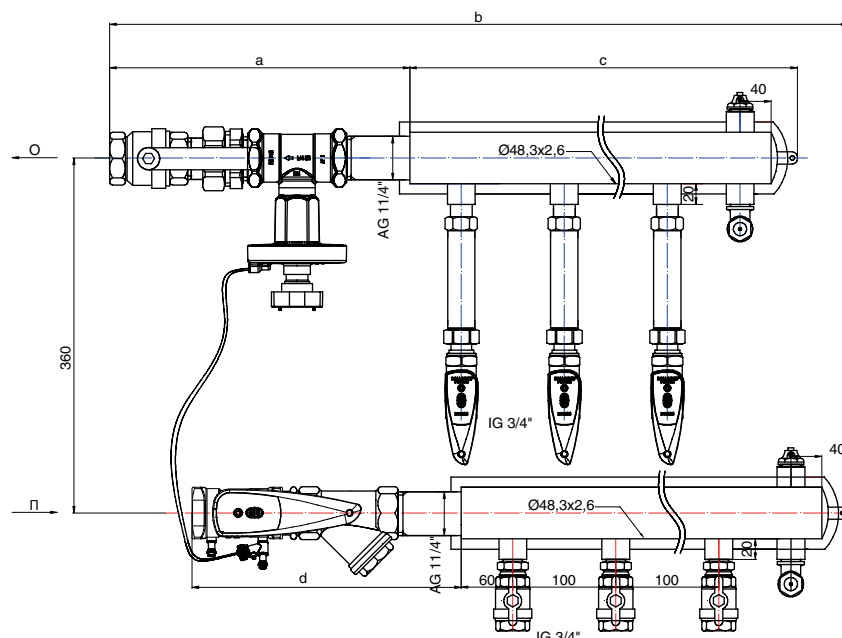
ПРИНЦИПИАЛЬНАЯ СХЕМА
