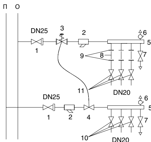
ПРИНЦИПИАЛЬНАЯ СХЕМА
