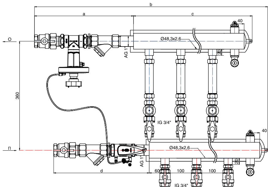
ПРИНЦИПИАЛЬНАЯ СХЕМА
