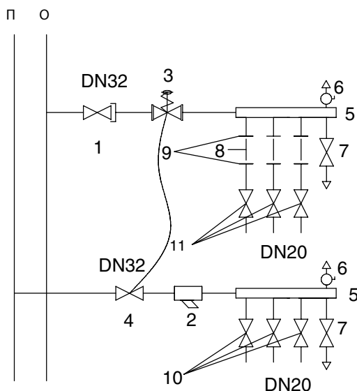
ПРИНЦИПИАЛЬНАЯ СХЕМА
