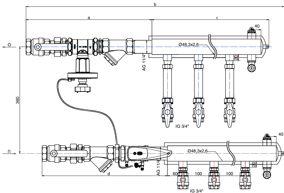
ПРИНЦИПИАЛЬНАЯ СХЕМА
