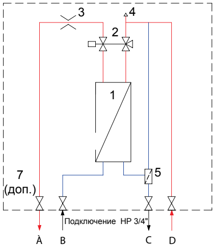
СХЕМА №1 (БАЗОВАЯ КОМПЛЕКТАЦИЯ)
