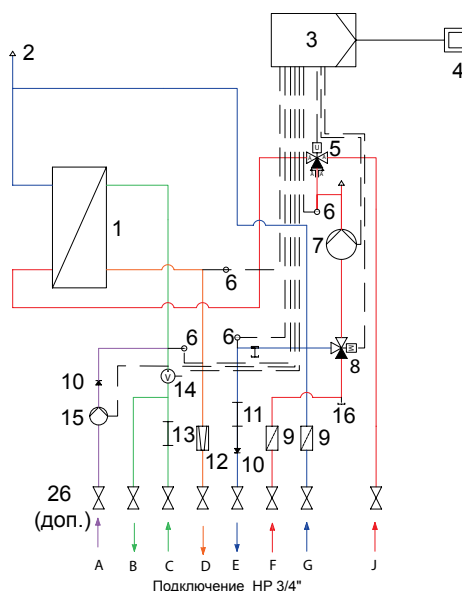
СХЕМА №1 (БАЗОВАЯ КОМПЛЕКАЦИЯ)
