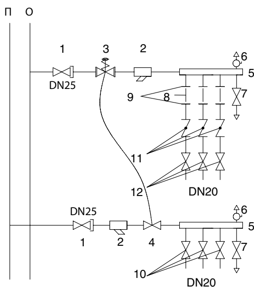
ПРИНЦИПАЛЬНАЯ СХЕМА
