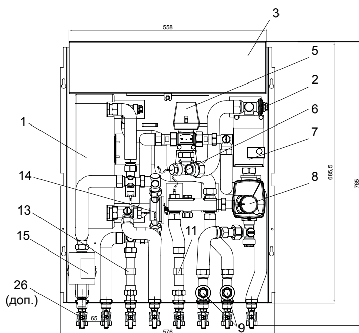
СХЕМА №1 (БАЗОВАЯ КОМПЛЕКАЦИЯ)
