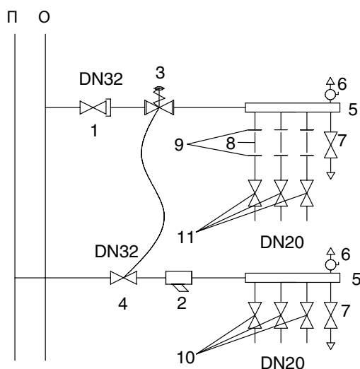
ПРИНЦИПИАЛЬНАЯ СХЕМА
