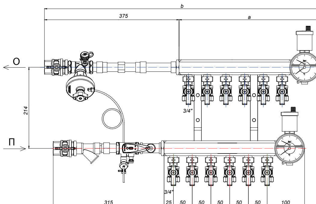
ПРИНЦИПИАЛЬНАЯ СХЕМА
