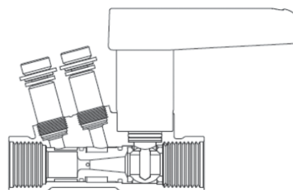
Конструкция клапана Meibes Ballorex Venturi FODRV
