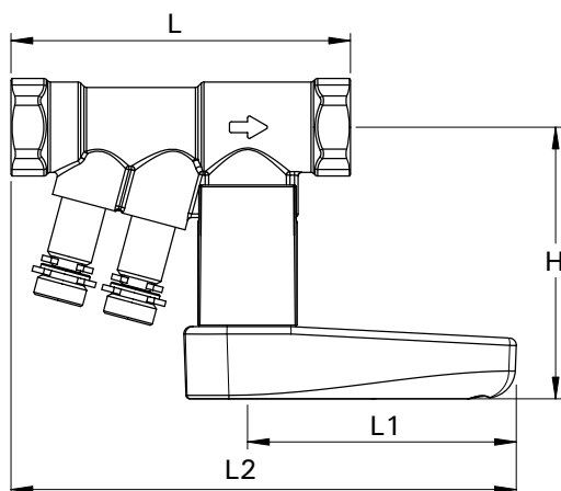
Размеры Ballorex Venturi FODRV с 2 измерительными ниппелями
