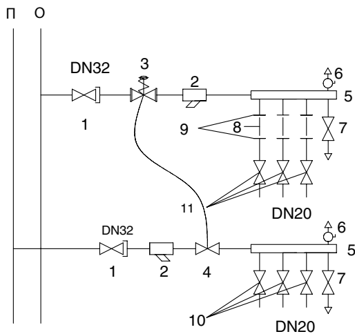
ПРИНЦИПИАЛЬНАЯ СХЕМА
