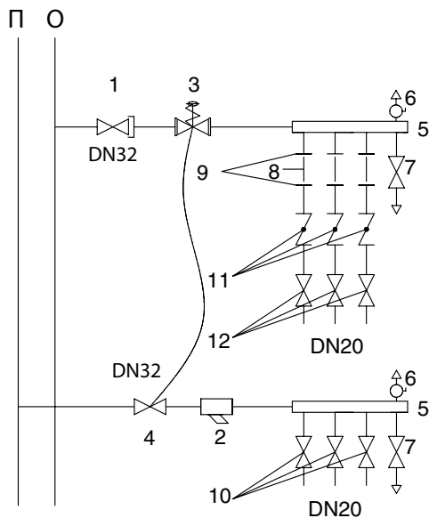
ПРИНЦИПИАЛЬНАЯ СХЕМА
