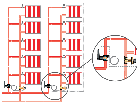
Ballorex Vario вне регулируемого контура
