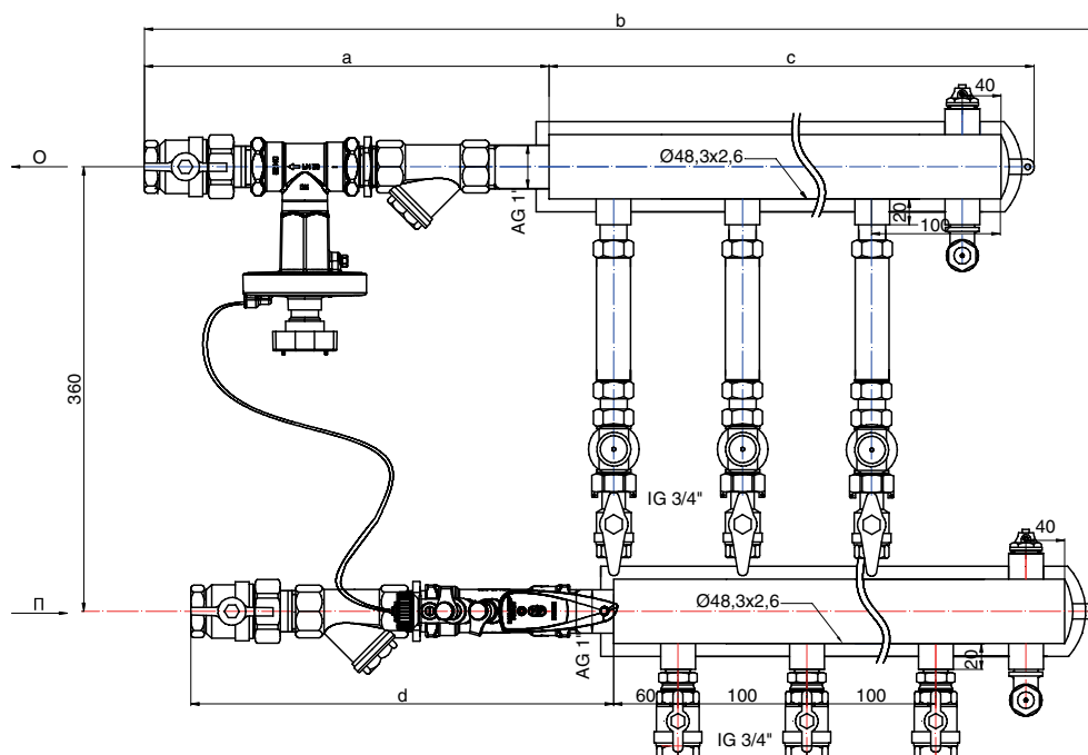
ПРИНЦИПИАЛЬНАЯ СХЕМА
