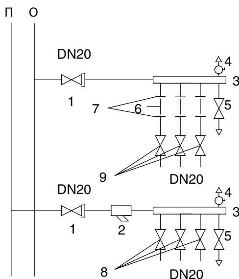
ПРИНЦИПИАЛЬНАЯ СХЕМА
