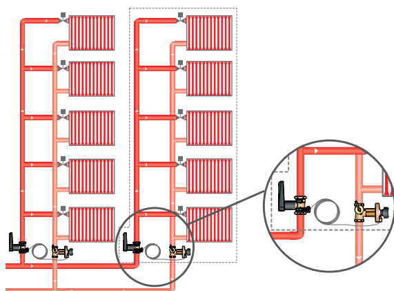
Ballorex Vario внутри регулируемого контура
