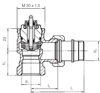
Термостатический клапан угловой с внутренней резьбой
