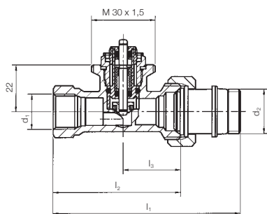
Термостатический клапан проходной с внутренней резьбой
