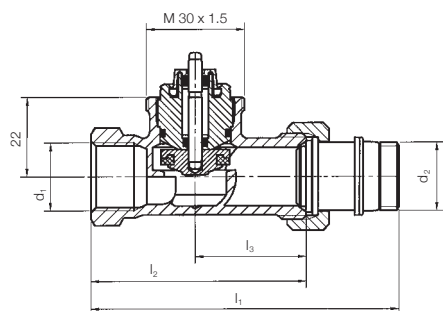
Термостатический клапан проходной с внутренней резьбой
